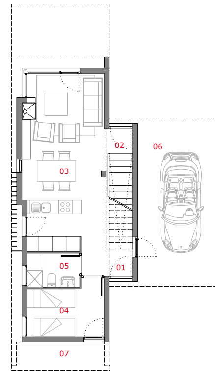
Planta Baixa
