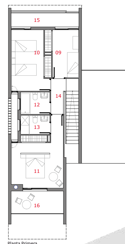
Planta Primera
