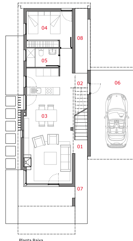
Planta Baixa
